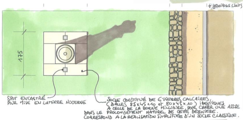
Dessin de détail des bornes milliaires
