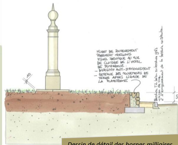
Dessin de détail des bornes milliaires
