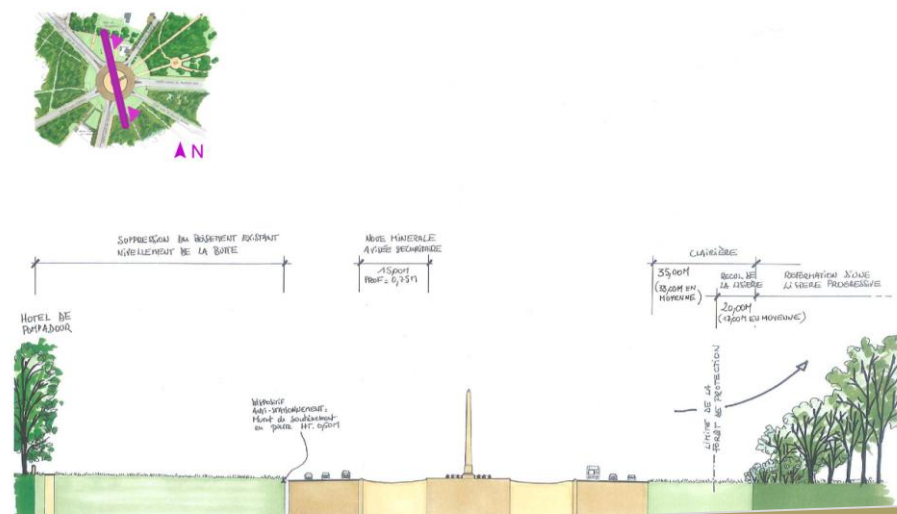
Coupe sur le carrefour de l'Obélisque
